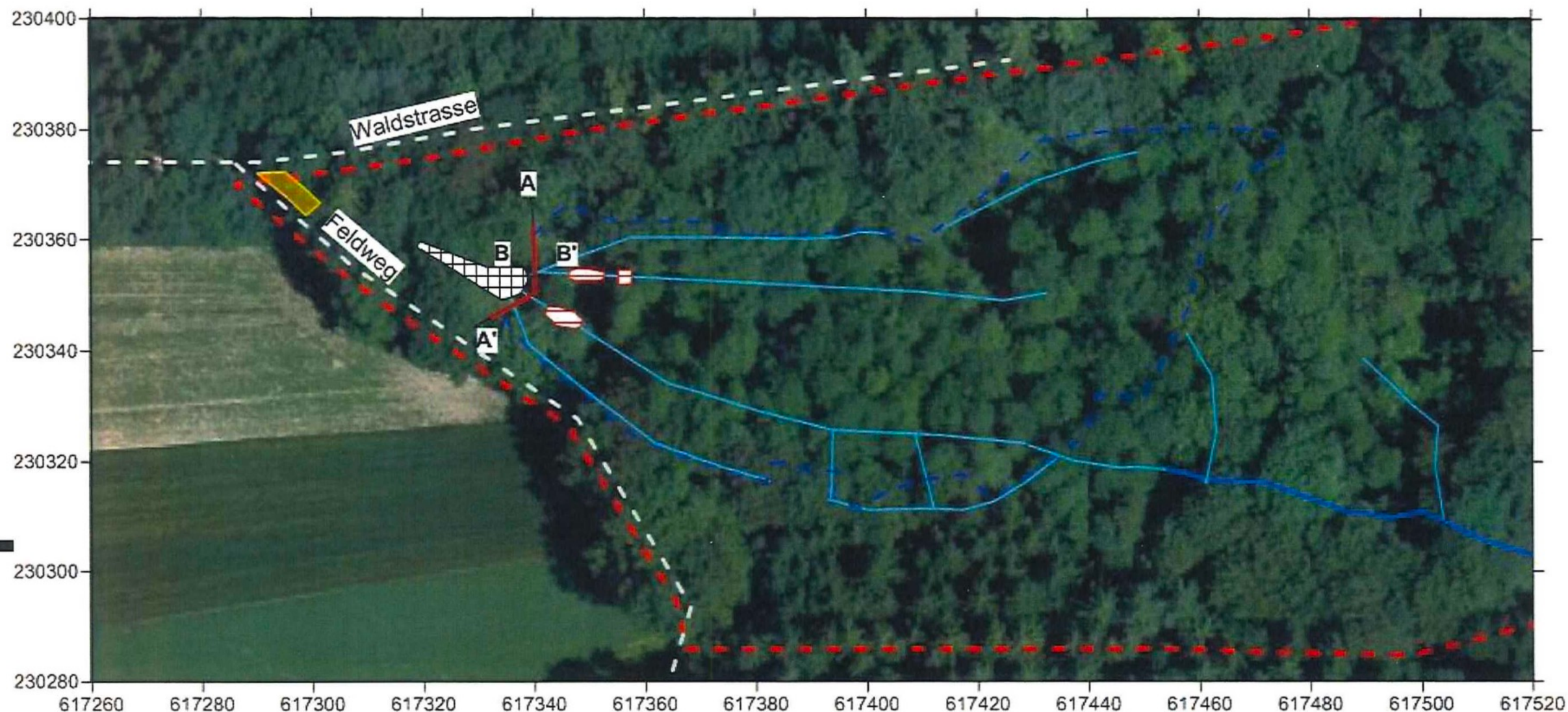
Abb. 1: Massnahmenplan vor aktuellem Luftbild. Ergänzend dargestellt ist die Versickerungsfläche am Westende des Dägimmooses sowie das zuführende Grabensystem. Die zu den Schnittlinien A und B zugehörigen Schnitte sind in der Beilage «Längs- und Querschnitt Spundwand» ersichtlich. Ebenfalls sichtbar ist der Bereich, der durch die Massnahmen stark vernässt wird.
